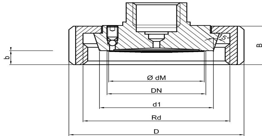
Somun Bağlantılı Konik Yataklamalı PN 40 bar
