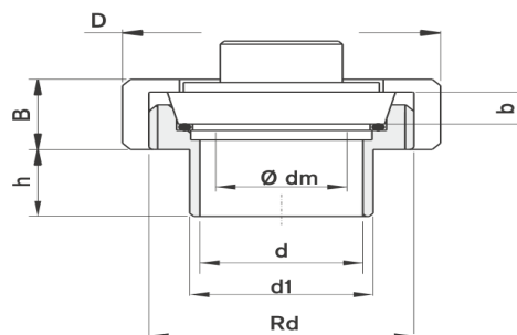
Kaynak Boyunlu Rakorlu Konik Yataklamalı PN 40 bar
