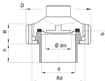
Kaynak Boyunlu Somunlu Konik Yataklamalı PN 40 bar
